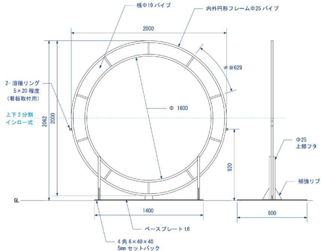
フレーム土台サイズ
